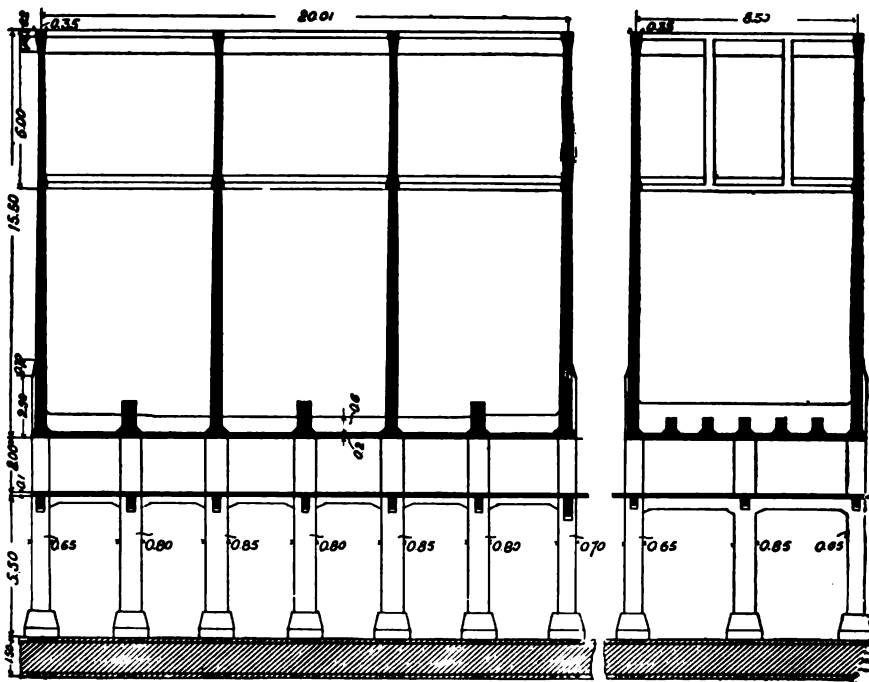
FIG. 325.—Välklingen coal pockets.
