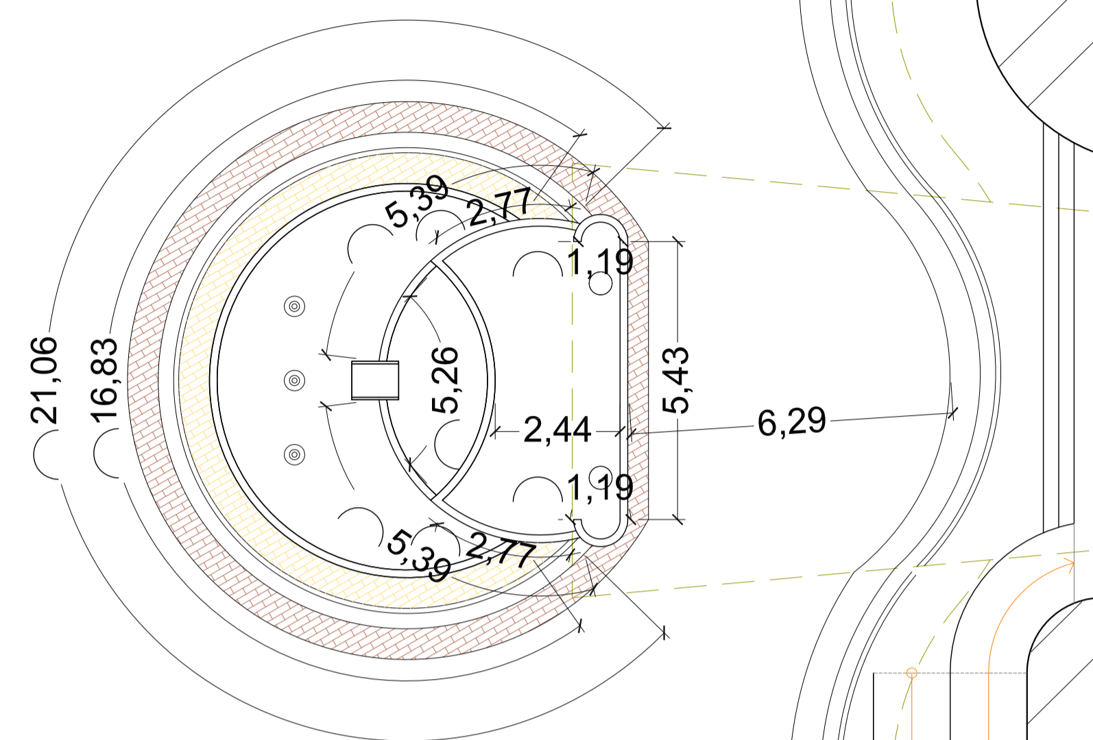
DETALHE CHAFARIZ DIMENSÕES COM COTAS GERAIS
